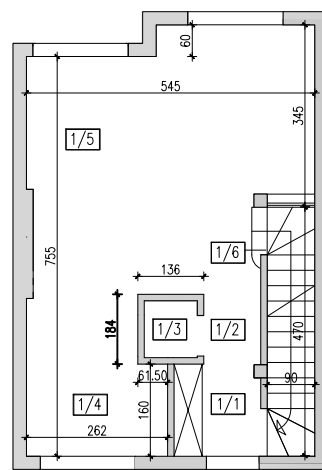
WYKAZ POMIESZCZEŃ SEGMENTU A5
