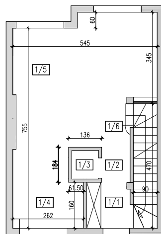
WYKAZ POMIESZCZEŃ SEGMENTU A3
