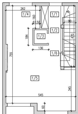
WYKAZ POMIESZCZEŃ SEGMENTU B5
